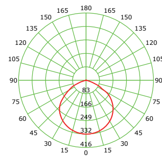
CURVA FOTOMETRICA
